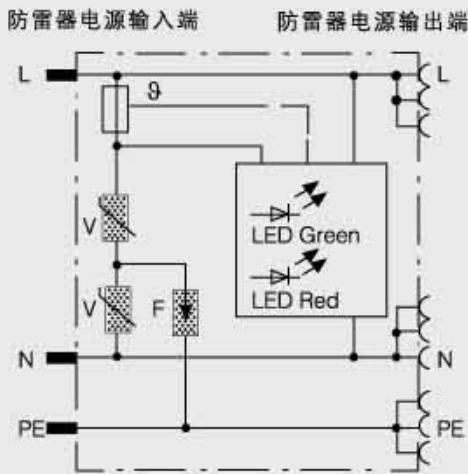
CNS 3-D-PRC结构图
