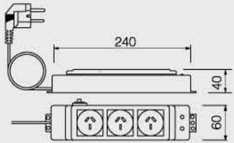
CNS 3-D-PRC尺寸图
